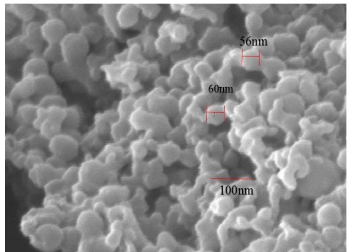
شکل ۵ ویژگی‌های ریخت‌شناسی نانوذرات اگزالی‌پالادیم با استفاده از میکروسکوپ الکترونی روبشی
